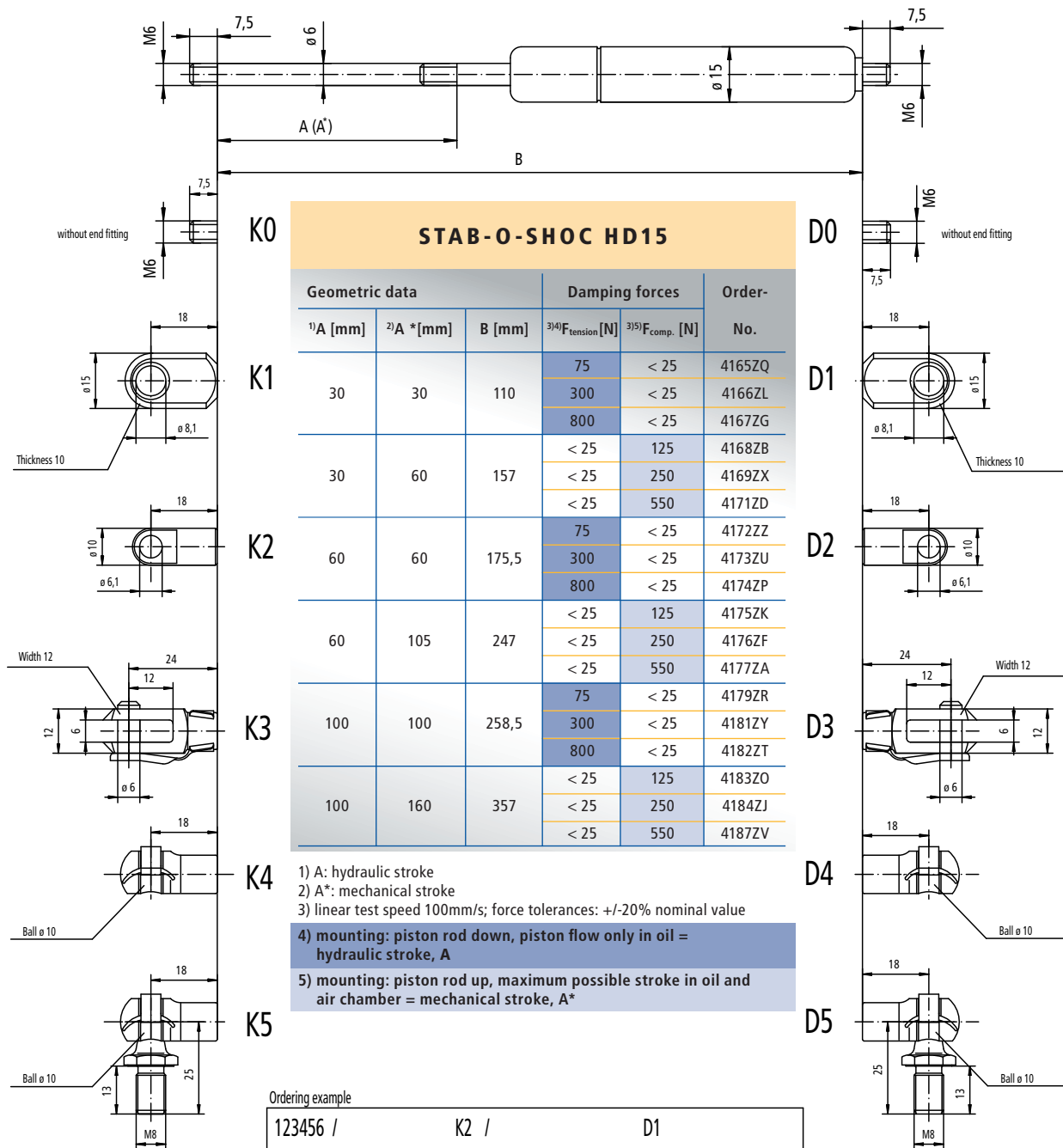
eyelet D1
